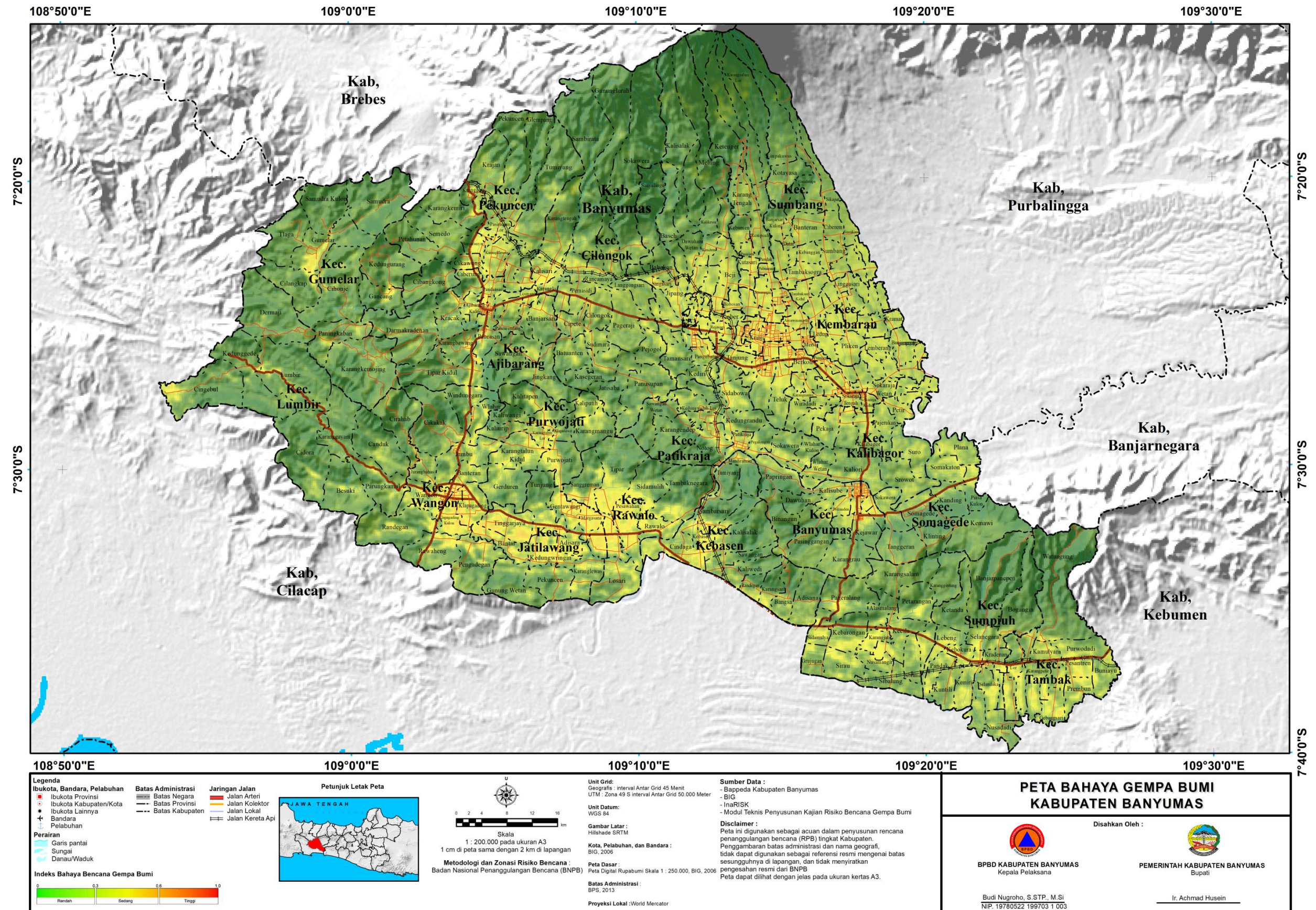
Gambar 7. Peta Bahaya Gempa Bumi Kabupaten Banyumas
