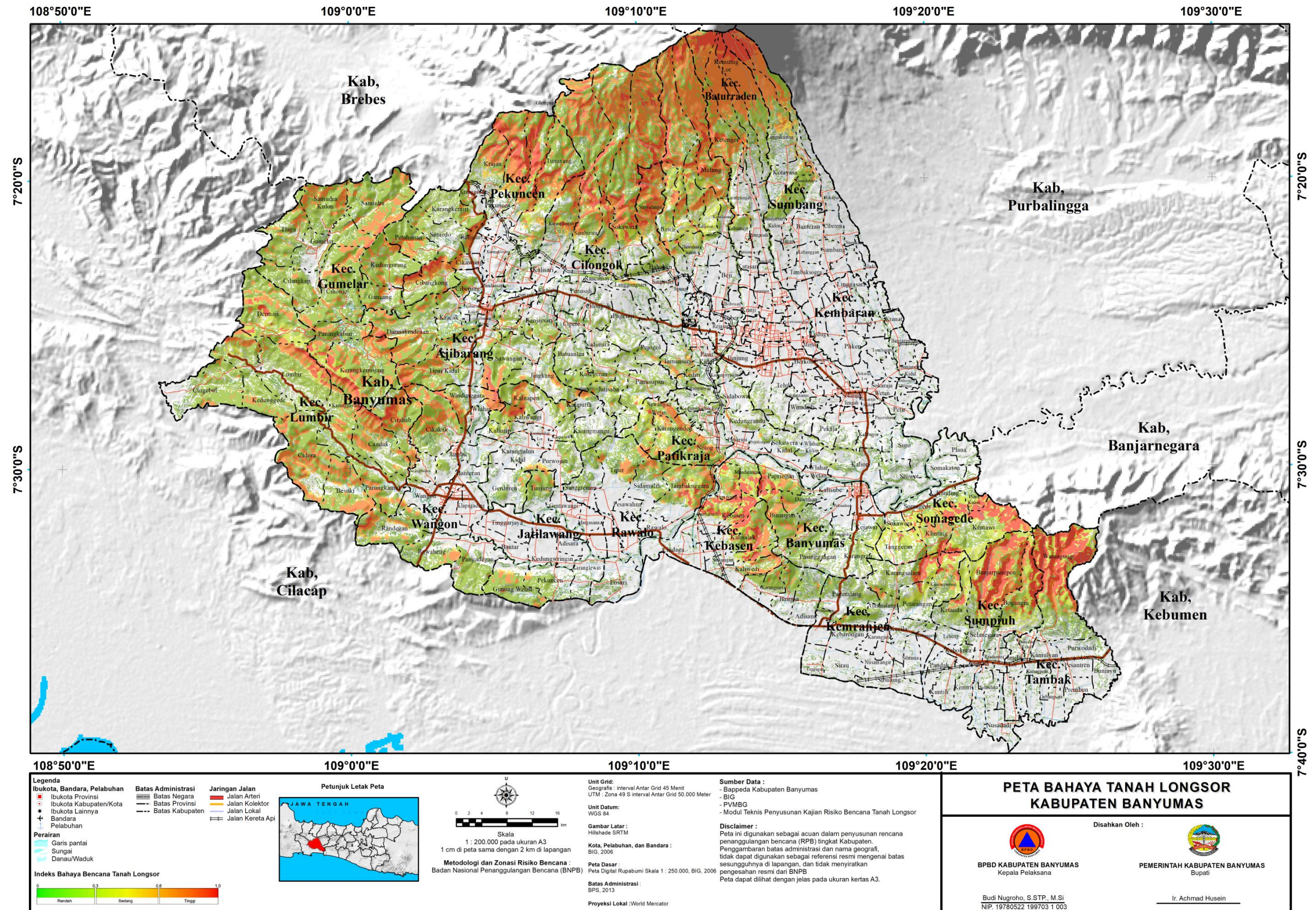
Gambar 6. Peta Bahaya Tanah Longsor Kabupaten Banyumas
