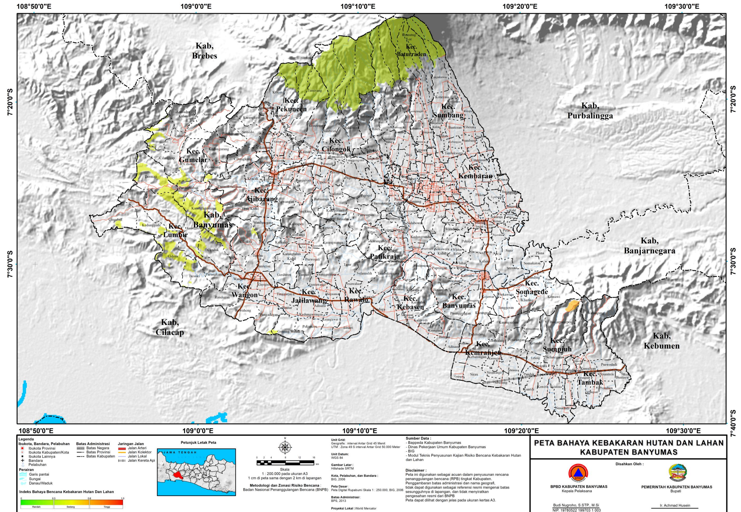
Gambar 8. Peta Bahaya Kebakaran Hutan Dan Lahan Kabupaten Banyumas
