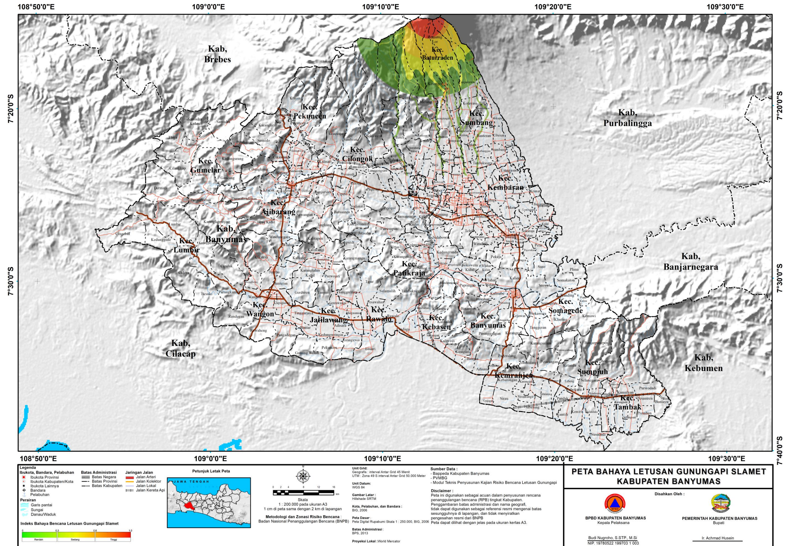
Gambar 9. Peta Bahaya Letusan Gunungapi Slamet Kabupaten Banyumas
