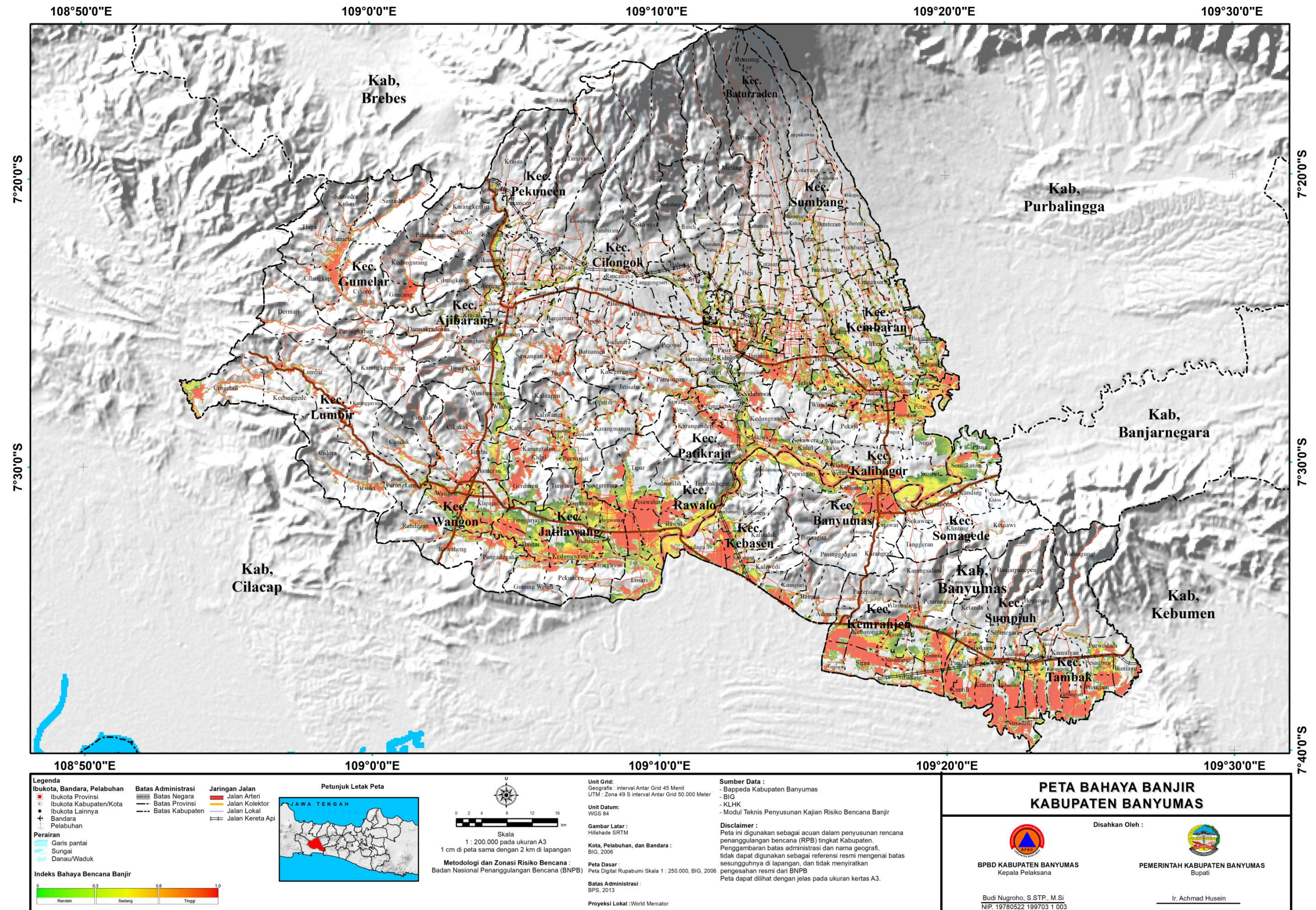
Gambar 3. Peta Bahaya Banjir Kabupaten Banyumas
