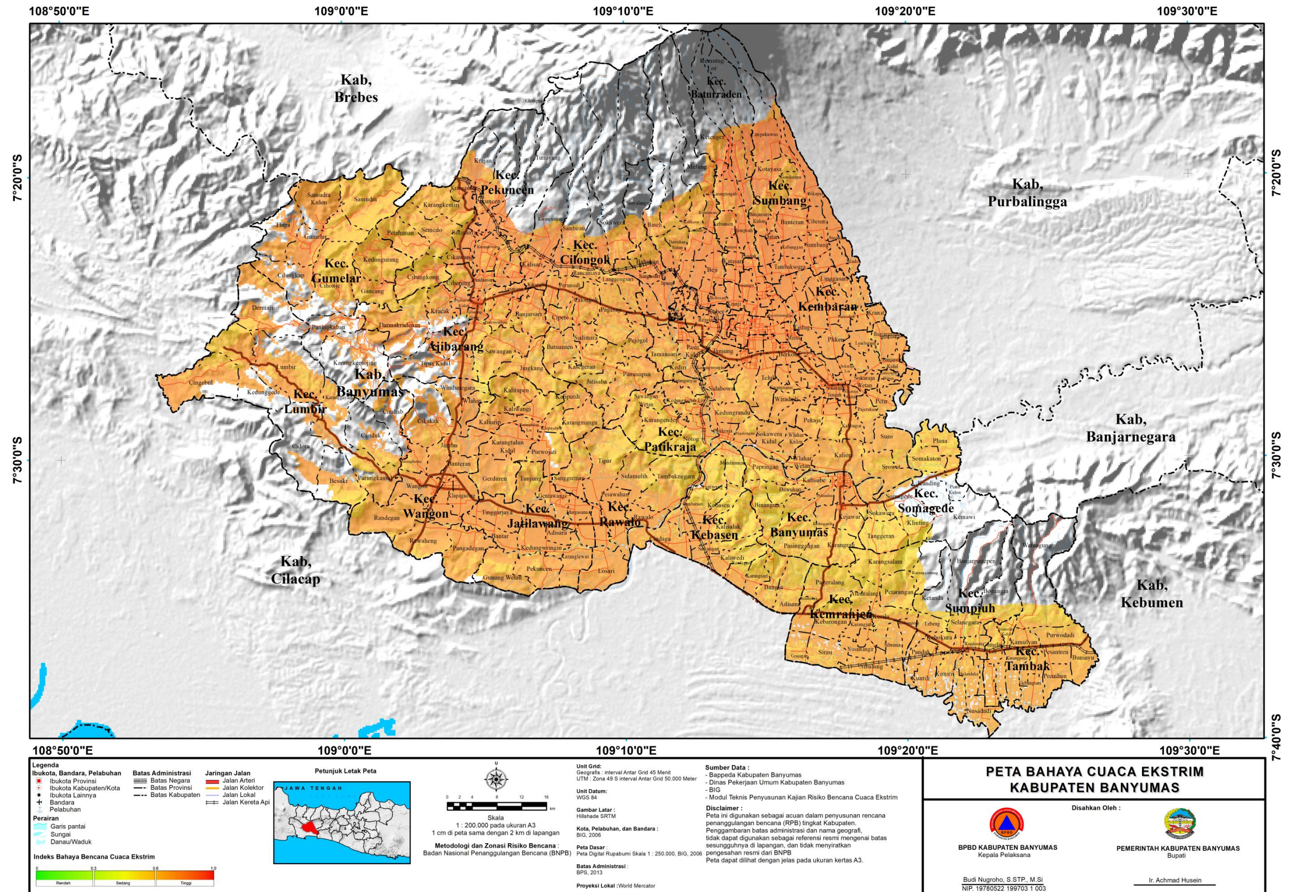
Gambar 4. Peta Bahaya Cuaca Eksreim Kabupaten Banyumas
