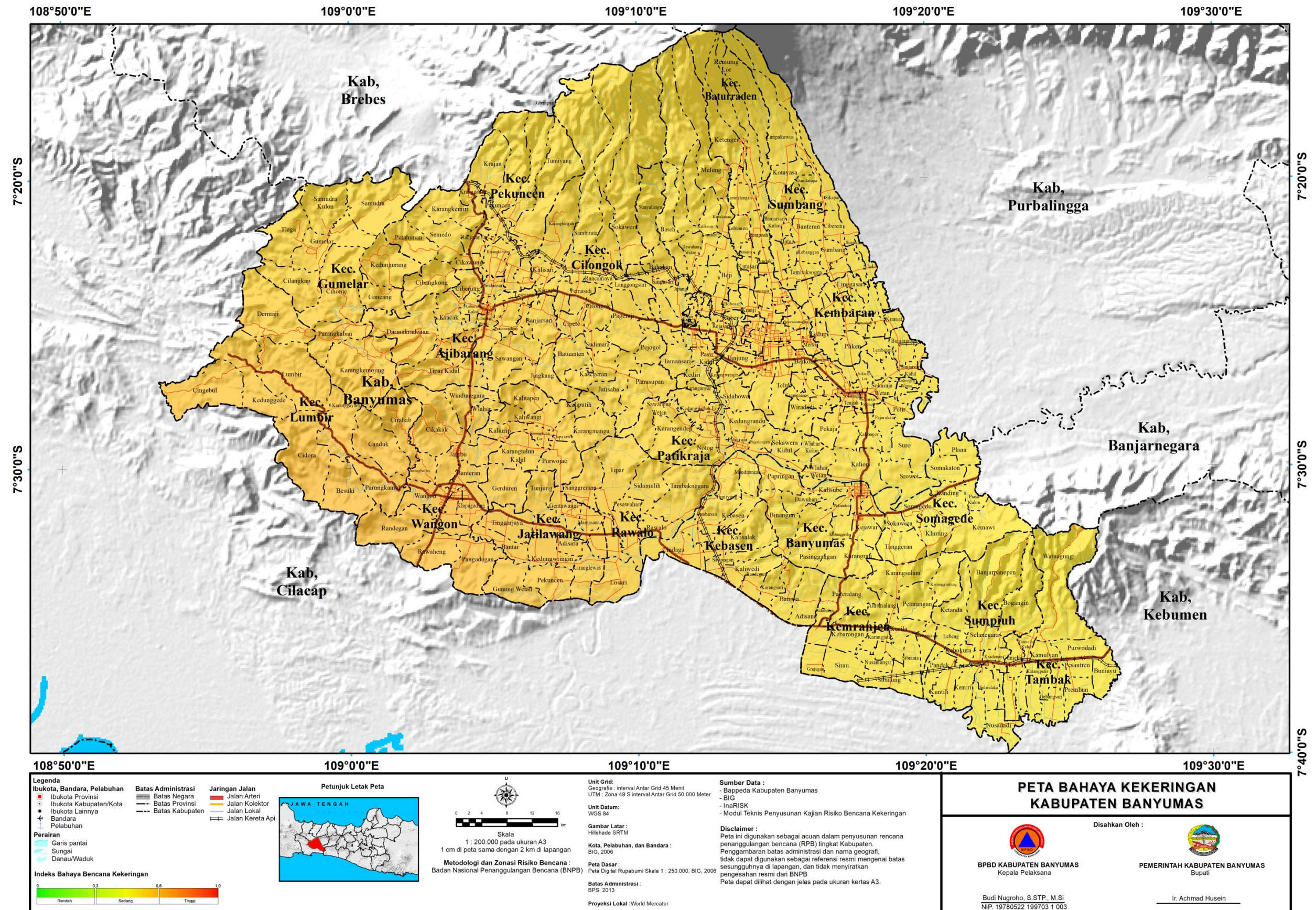
Gambar 5. Peta Bahaya Kekeringan Kabupaten Banyumas
